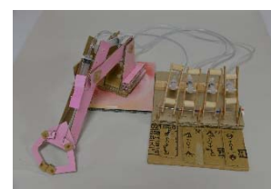
水圧ロボットアーム
